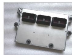
3408501 Electronic Control Module ECM 电脑模块
